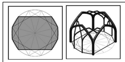
تصویر ۹: گسترش کاربردی از طریق امتداد تیر طاق‌ها در محدوده دایره محیطی ماخذ: محمدیان منصور و فرامرز، ۱۳۹۰.
