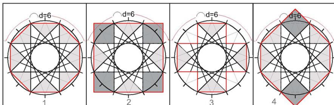
تصویر ۱۶: پیاده‌سازی کاربندی ۱۶ با هندسه مشخص و فاصله اتصال ثابت ( d=6 ) در زمینه‌های مختلف (۱- زمینه هشت ضلعی، ۲- زمینه مربع، ۳- زمینه چلیپا، ۴- زمینه شش ضلعی نامنتظم)، مأخذ: نگارندگان.
