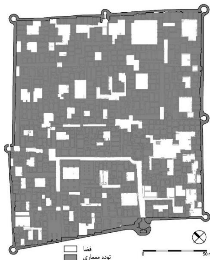
تصویر ۱۳: نقشه نولی از نظام توده - فضا در قلعه تاریخی مورچه‌خورت؛ فشردگی و تراکم سازمان شهری و اتصال بناها (مأخذ: نگارنده اول، ۱۴۰۰، باز طراحی بر اساس منوچهری، ۱۳۸۷: ۴۷).
