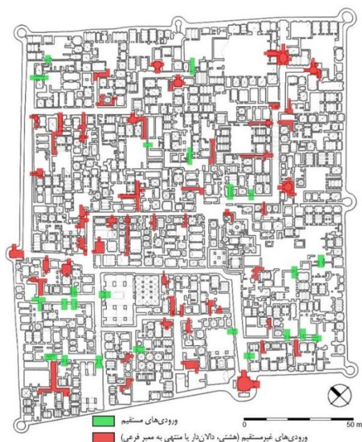
تصویر ۱۶: انواع ورودی در واحدهای معماری قلعه تاریخی مورچه‌خورت (مأخذ: نگارنده اول، ۱۴۰۰، باز طراحی بر اساس منوچهری، ۱۳۸۷: ۴۷)
