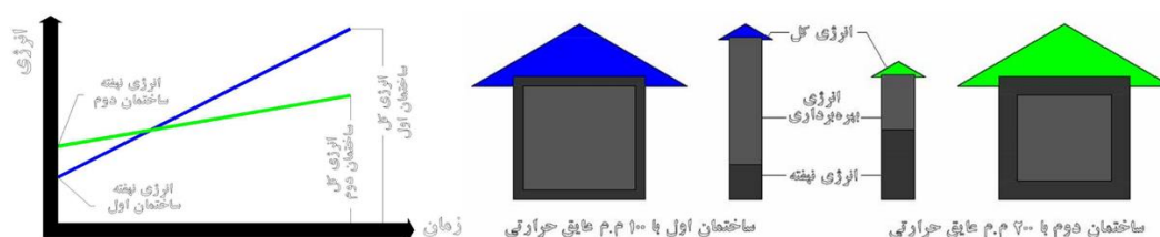
تصویر ۷: مقایسه تغییرات انواع انرژی در ساختمان با توجه به تغییر در میزان عایق حرارتی (مأخذ: (Menzies, 2011))
