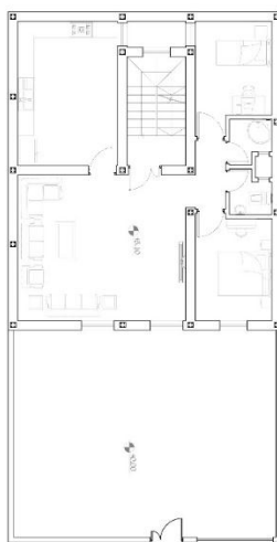
پلان طبقه اول
