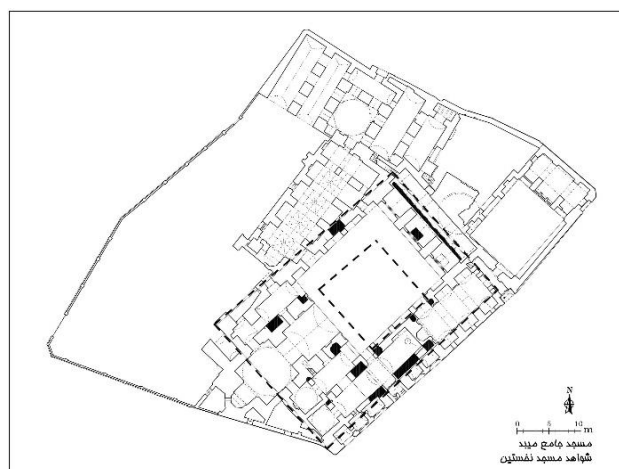
تصویر ۷: نقشه مسجد جامع میبد حدود و بقایای مسجد نخستین (مأخذ: نیک‌زاد، ۱۳۹۵، ۱۱۸، به‌روزرسانی و افزوده‌ها از نگارنده).
