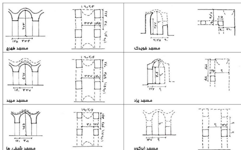
تصویر ۳۸: اندازه‌ها و تناسبات فضای شبستان در مقطع افقی و عمودی مساجد (ترسیم از نگارنده).
